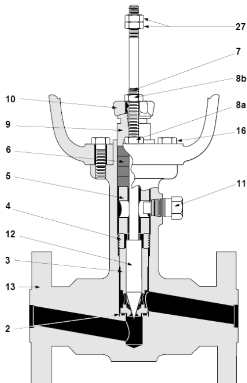
Регулятор серии 535V
